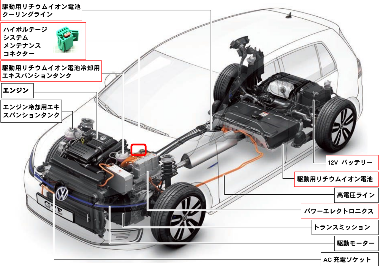
駆動用リチウムイオン電池 (赤枠は作業か所)
