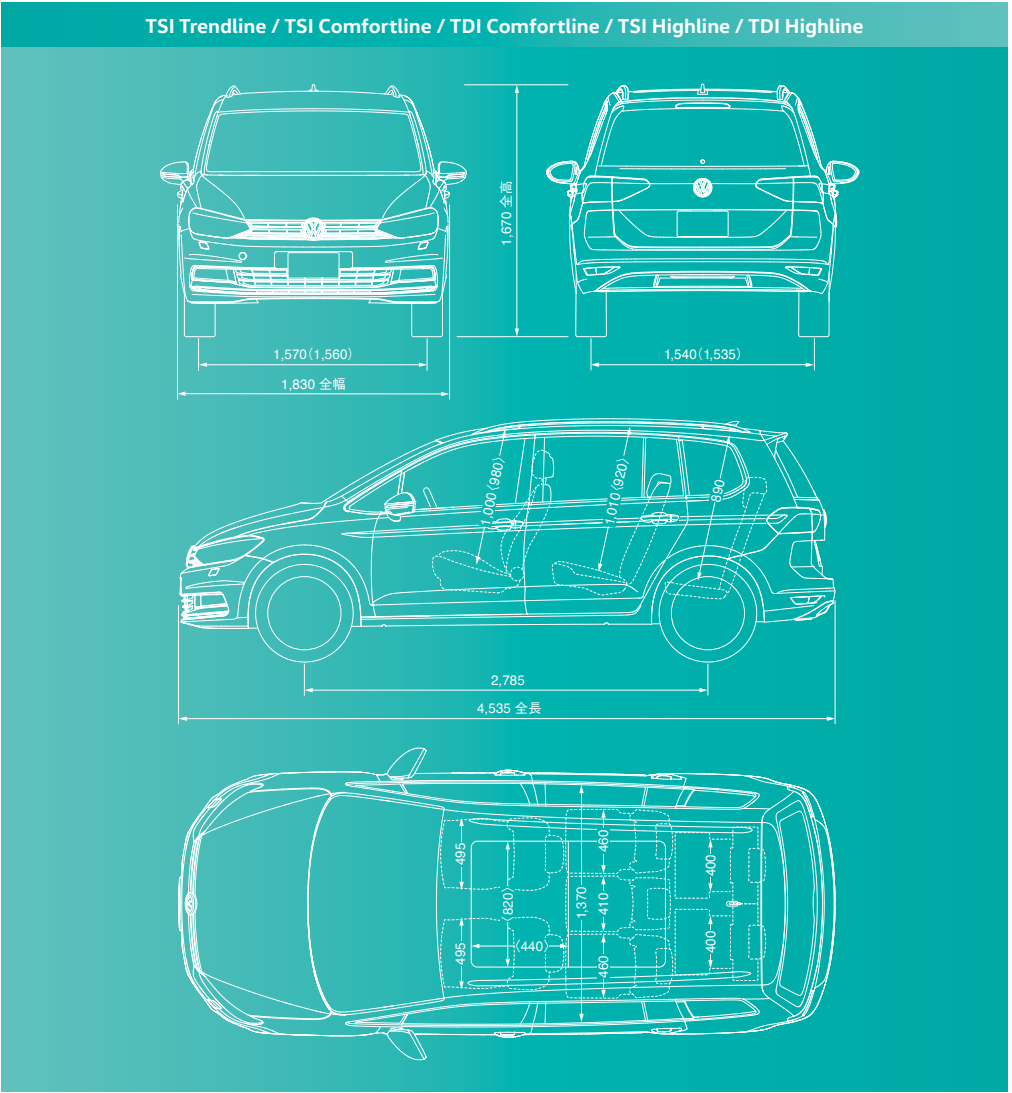
四面図(mm)
