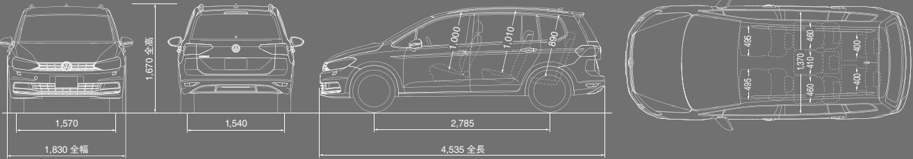
四面図 (mm)
