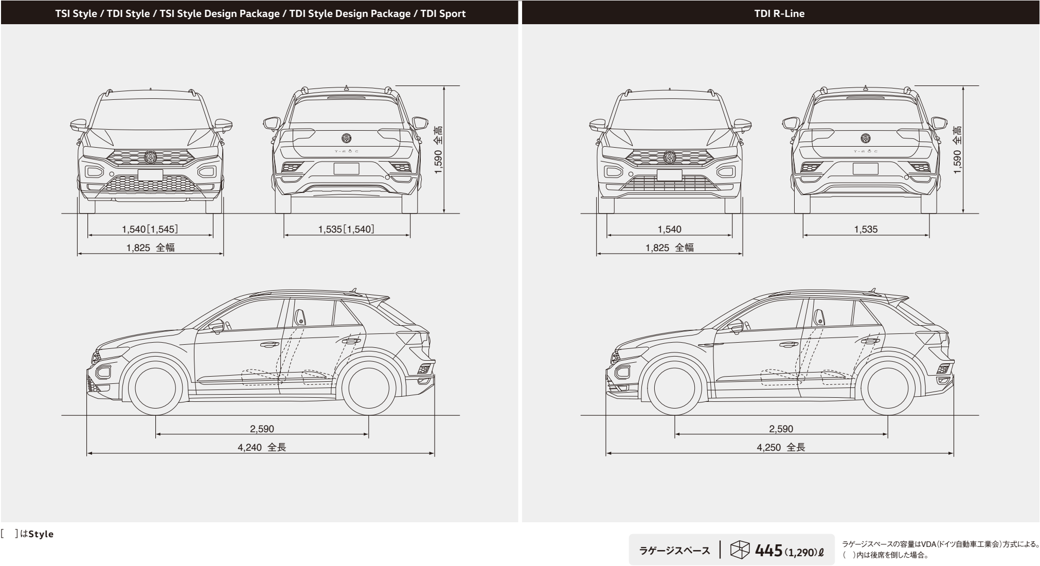
三面図 (mm)
