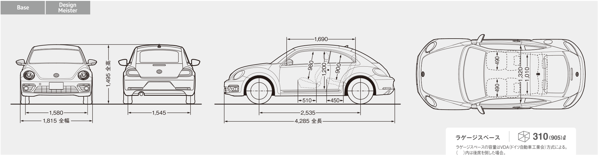
四面図(mm)
